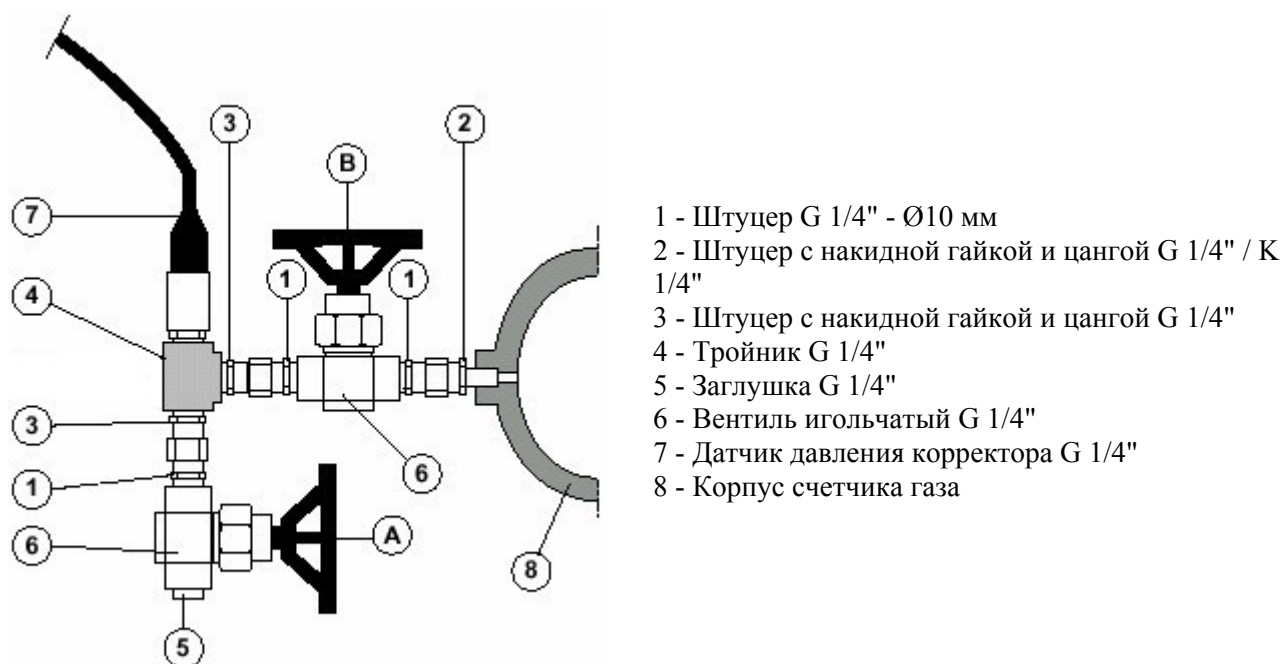
Рис. 4. Монтаж датчика давления при помощи монтажного комплекта
