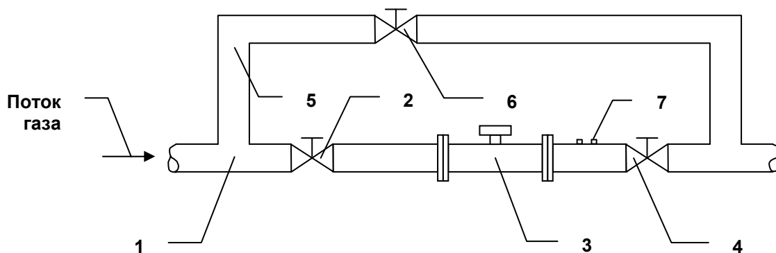
Рис. 2. Установка счетчика без перепускного канала
