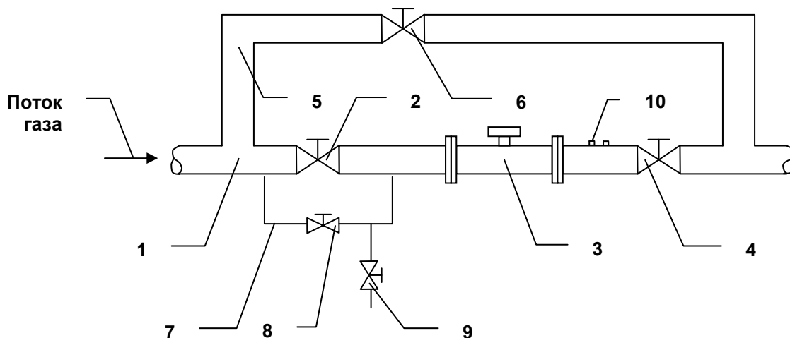
Рис. 3. Установка счетчика с перепускным каналом
