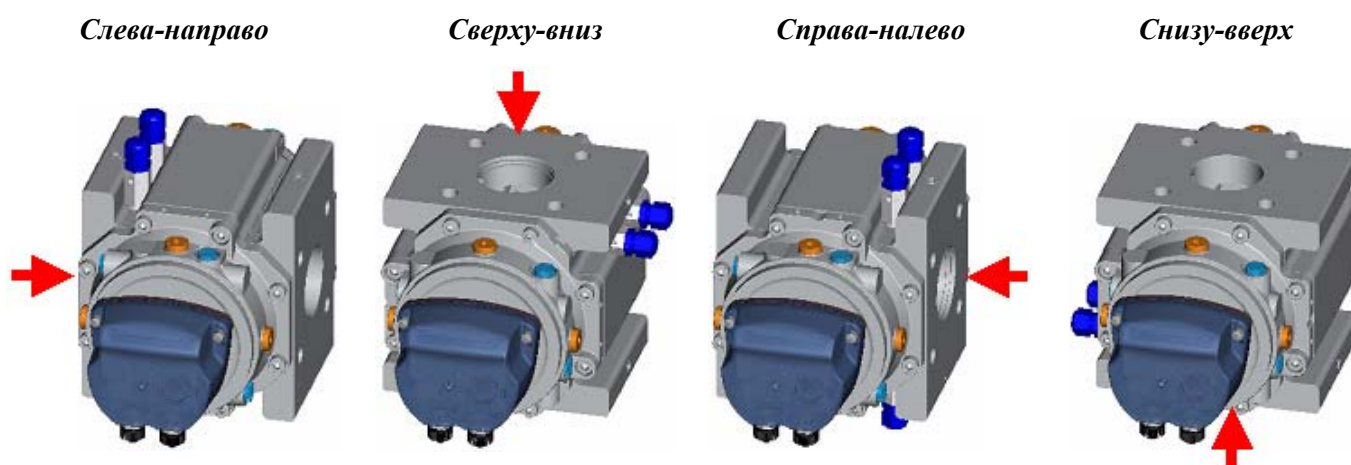
Рис. 3. Варианты установки счетчиков в зависимости от направления потока газа
