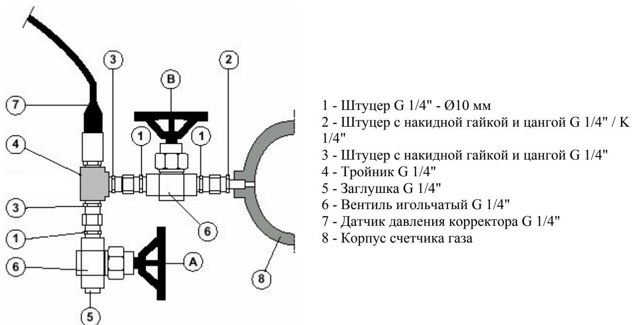
Рис. 7. Монтаж датчика давления при помощи монтажного комплекта
